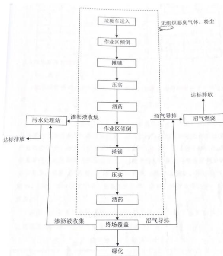
图3.3-1 生产工艺图
